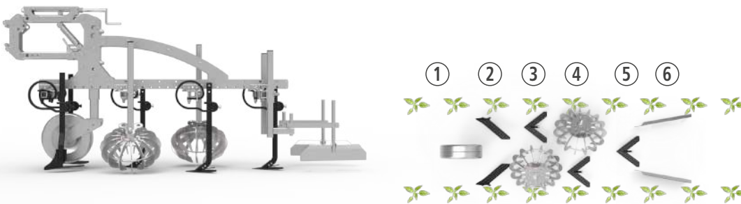
ELEMENTO ROTOSARK INTERFILAS con accesorios TRABAJO EN EL ESPACIO ENTRE FILAS
