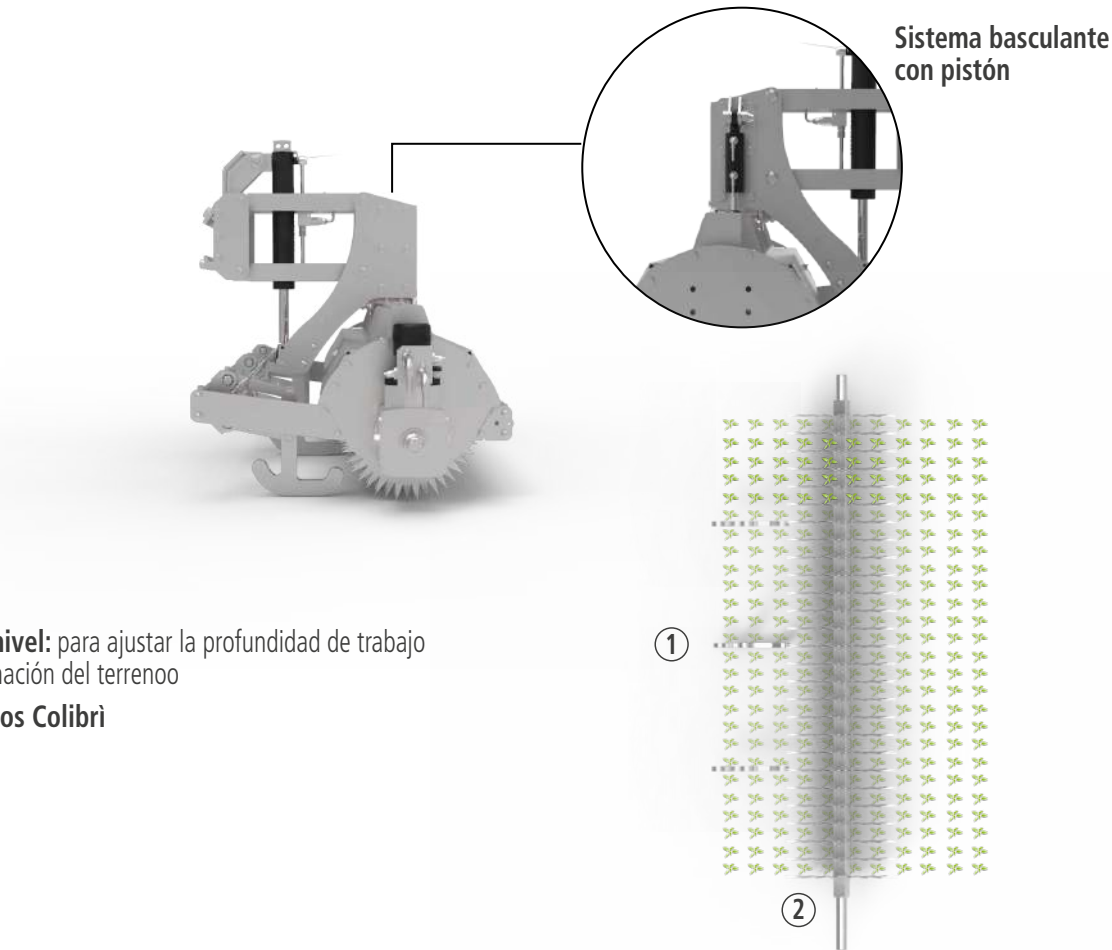
ELEMENTO COLIBRÌ BASCULANTE TRABAJO SOBRE LAS FILAS
